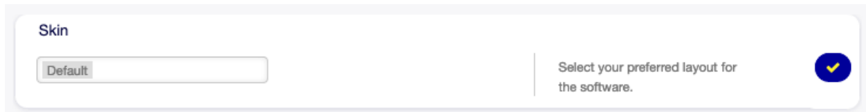
Fig. 3.14: Skin Widget
