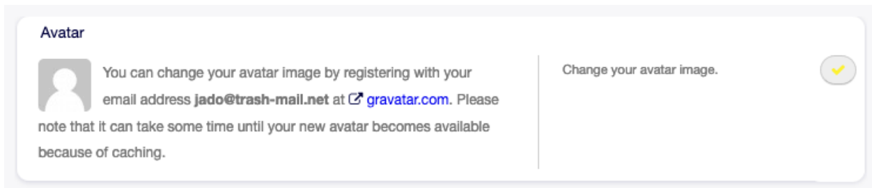
Fig. 3.5: Avatar Widget
