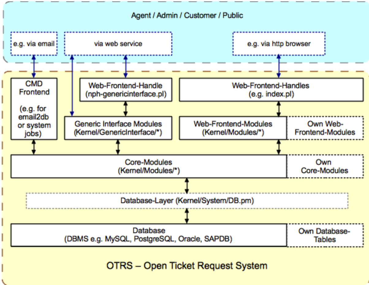
图 1: OTRS 架构
